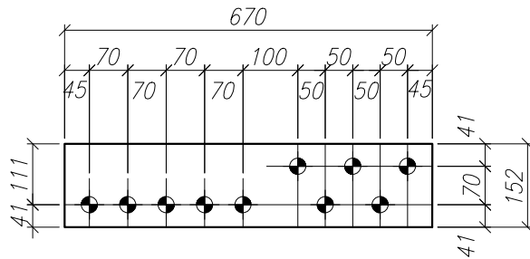
CUBREJ. INT. CI-5 44 Can.6 44 – 1 –CH 9.5 CANT. 1 OBS: * LARGO – ANCHO * 670 * 152
