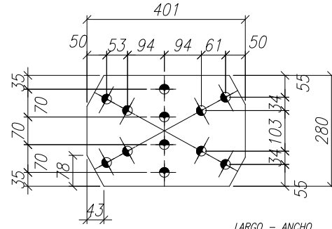
70 - 1 -CH 9.5 CANT. 1 OBS: LARGO - ANCHO * 401 * 280
