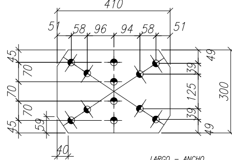
68 - 1 -CH 9.5 CANT. 1 OBS: LARGO - ANCHO * 410 * 300
