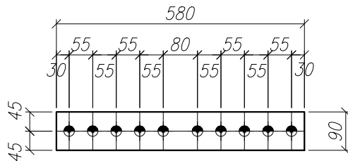
CUBREJ. INT. CI-7 46 Can.6 46 – 1 –CH 9.5 CANT. 1 OBS: * LARGO – ANCHO * 580 * 90
