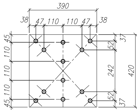
62 - 1 -CH 9.5 CANT. 1 OBS: LARGO - ANCHO * 420 * 390
