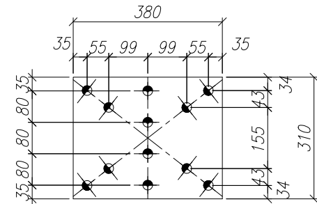
66 - 1 -CH 9.5 CANT. 1 OBS: LARGO - ANCHO * 380 * 310
