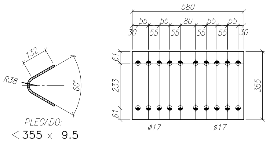
CUBREJ. EXT. C8 37 Can.3
