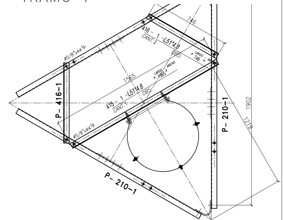
CUADRO TRAMO 10 CORTE K-K
