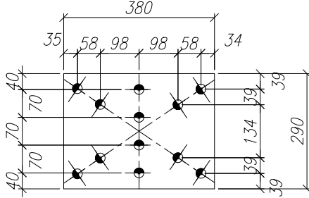
67 - 1 -CH 9.5 CANT. 1 OBS: LARGO - ANCHO * 380 * 290
