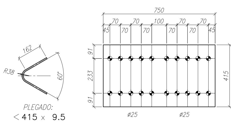
CUBREJ. EXT. C7 36 Can.3
