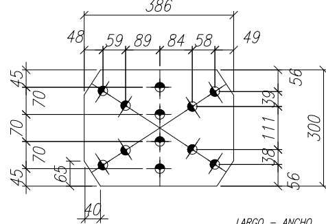
69 - 1 -CH 9.5 CANT. 1 OBS: LARGO - ANCHO * 386 * 300
