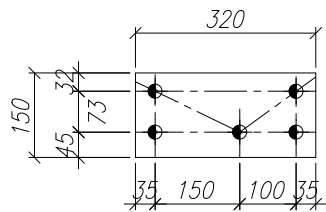
75 - 1 -CH 7.9 CANT. 1 OBS: LARGO - ANCHO * 320 * 150
