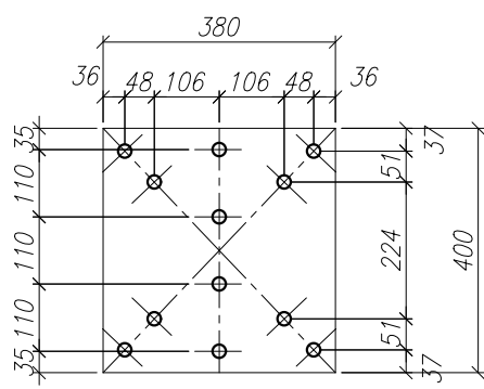
63 - 1 -CH 9.5 CANT. 1 OBS: LARGO - ANCHO * 400 * 380
