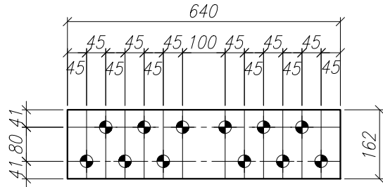
CUBREJ. INT. CI-3 42 Can.6 42 – 1 –CH 7.9 CANT. 1 OBS: * LARGO – ANCHO * 640 * 162
