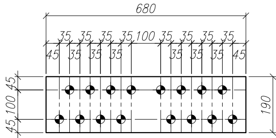
CUBREJ. INT. CI-1 40 Can.12 40 – 1 –CH 9.5 CANT. 1 OBS: * LARGO – ANCHO * 680 * 190
