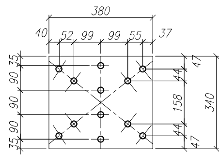
65 - 1 -CH 9.5 CANT. 1 OBS: LARGO - ANCHO * 380 * 340
