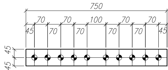
CUBREJ. INT. CI-6 45 Can.6 45 – 1 –CH 9.5 CANT. 1 OBS: * LARGO – ANCHO * 750 * 90
