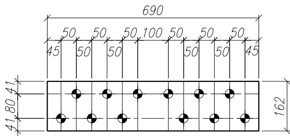
CUBREJ. INT. CI-4 43 Can.6 43 – 1 –CH 7.9 CANT. 1 OBS: * LARGO – ANCHO * 690 * 162
